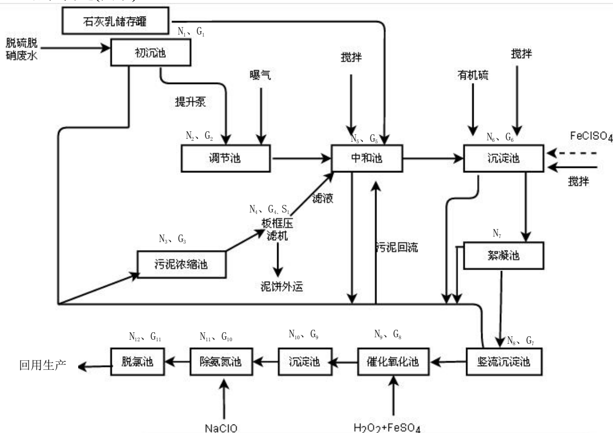
图 3 污水处理工艺流程及排污节点图
