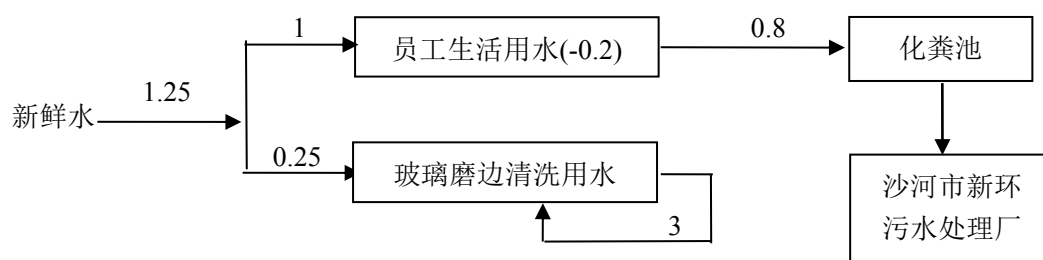
图 1 水量平衡图（单位： \text{m}^3/\text{d} ）
